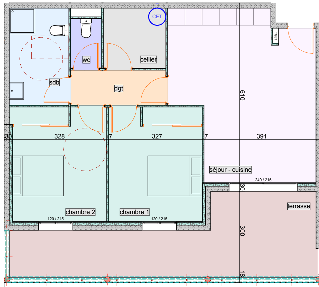
PLAN DE L'APPARTEMENT
