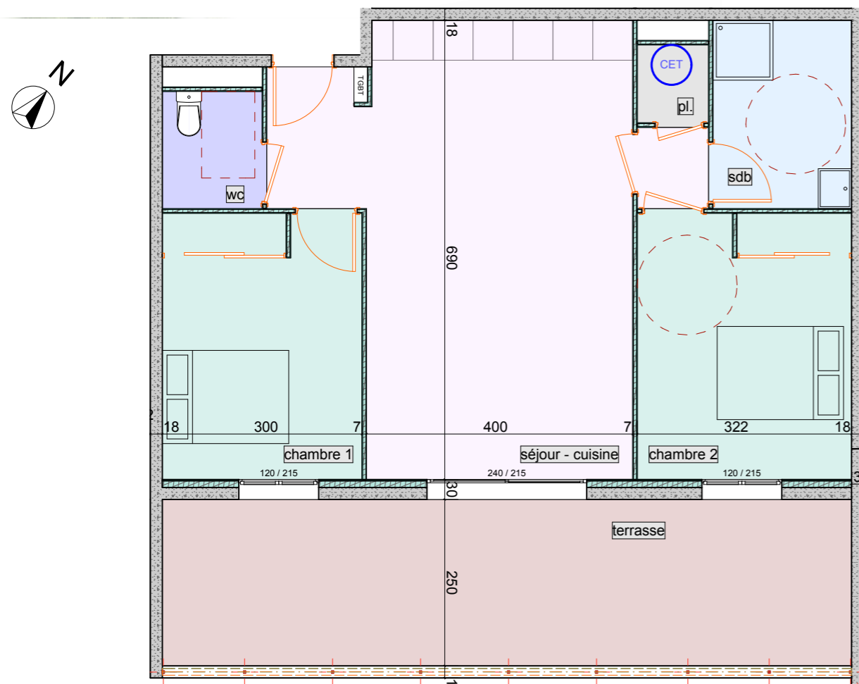
PLAN DE L'APPARTEMENT
