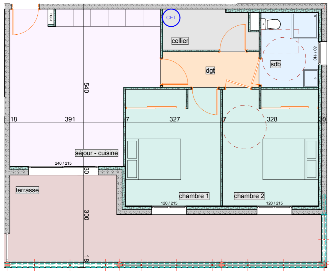
PLAN DE L'APPARTEMENT
