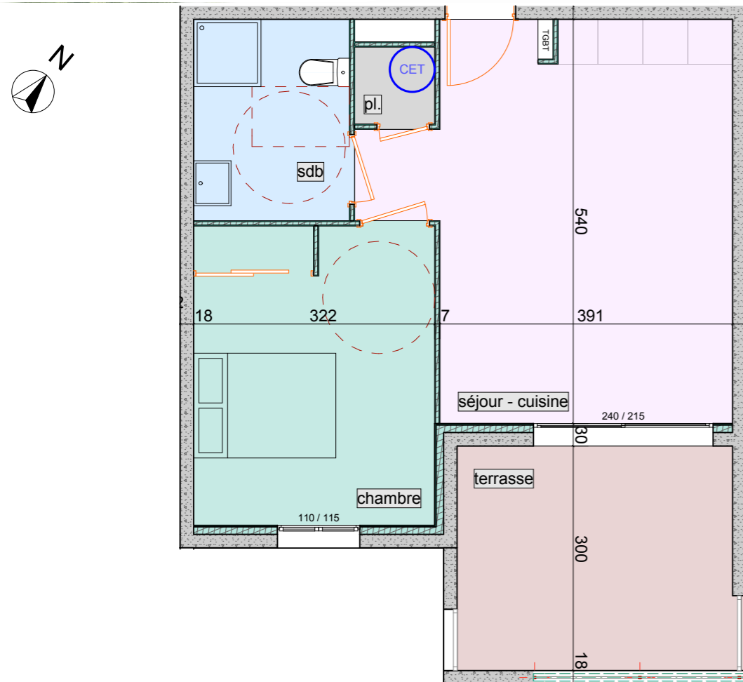
PLAN DE L'APPARTEMENT
